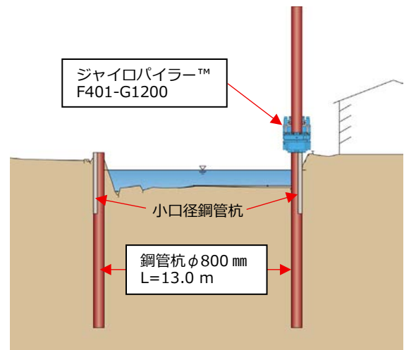
断面図
