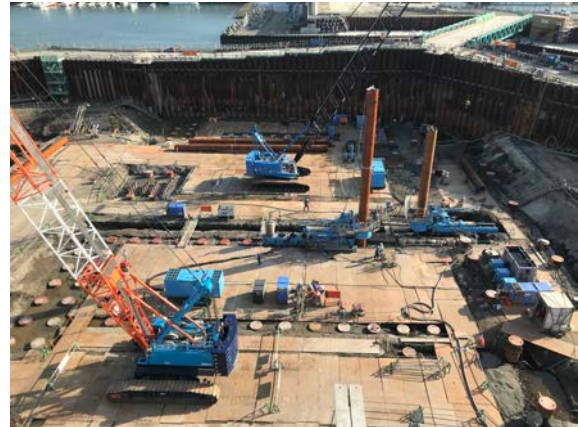
2017 年から 2 工区にわたり行われた水門基礎工事の様子
