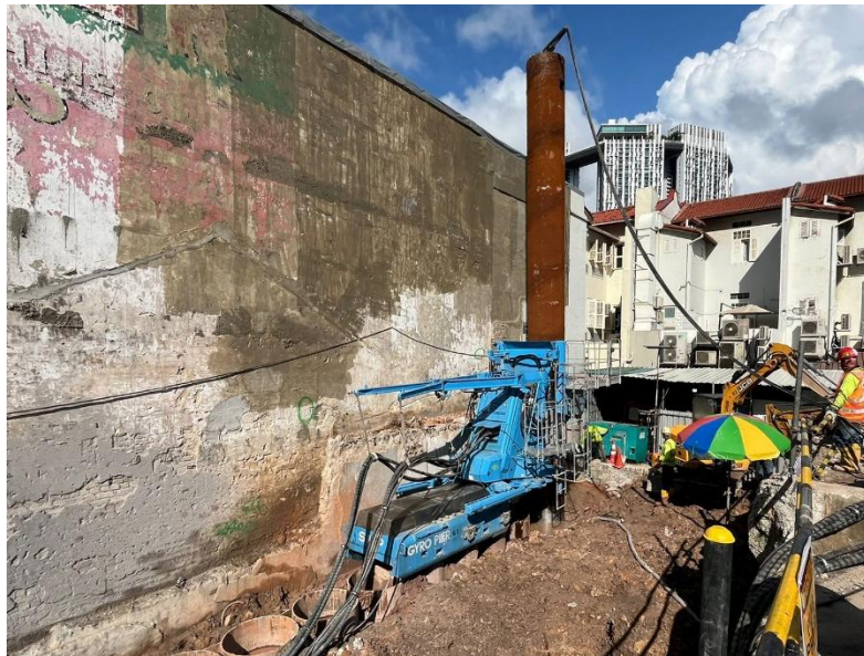
ジャイロプレス工法が採用されたホテル建設に伴う土留め工事
