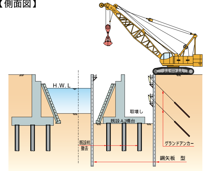
【側面図】
