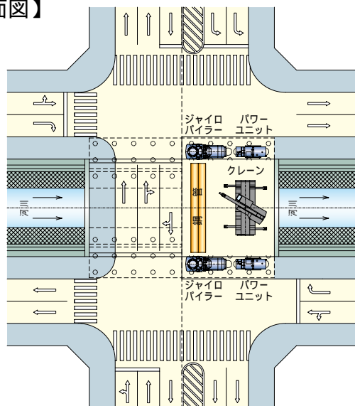
【平面図】
